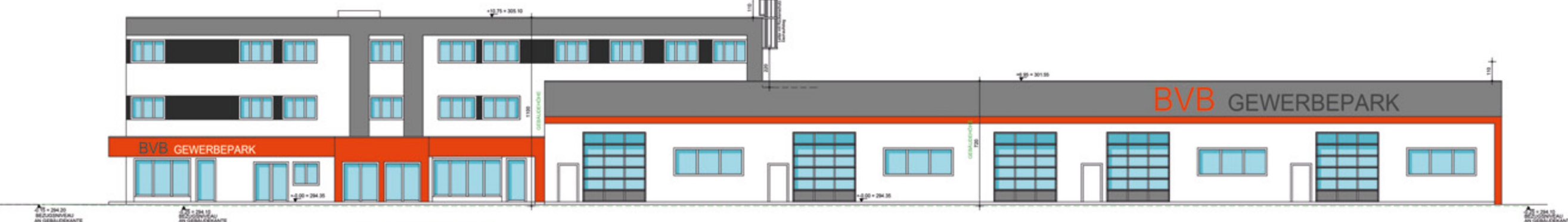
SÜD-OST ANSICHT
