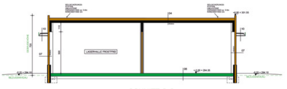
SCHNITT C-C
