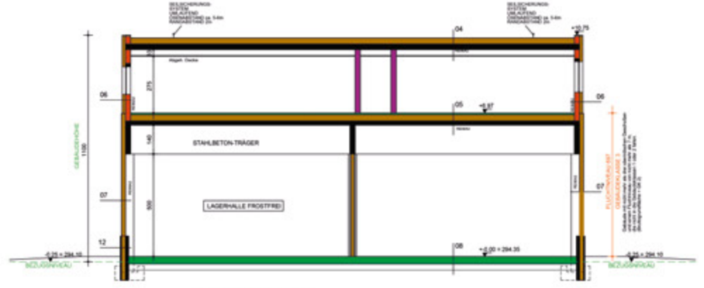
SCHNITT B-B
